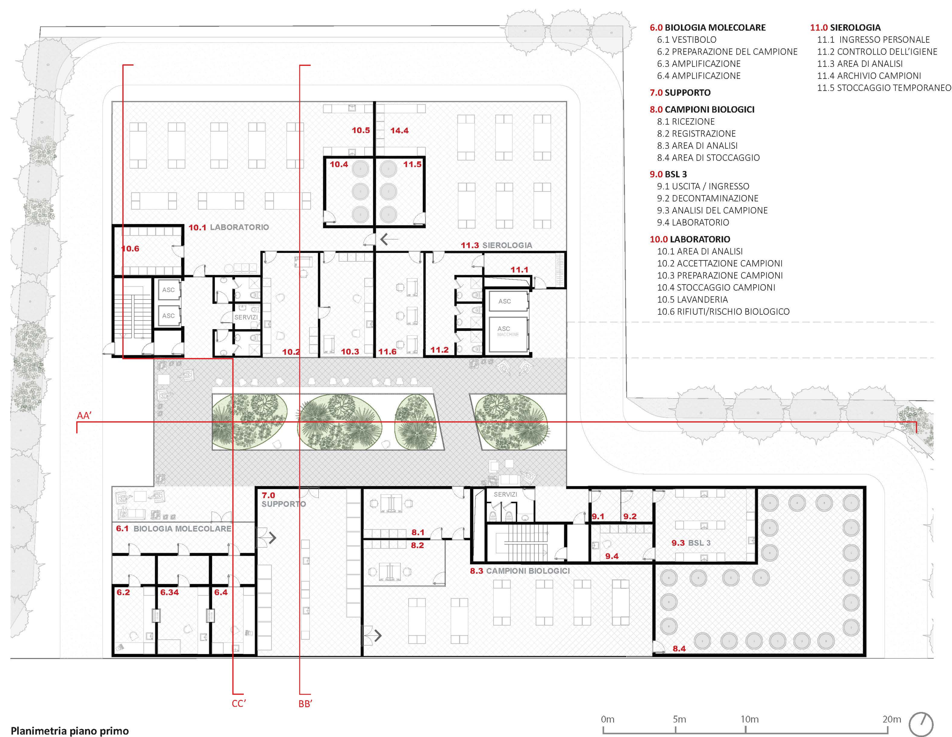
Planimetria piano primo
