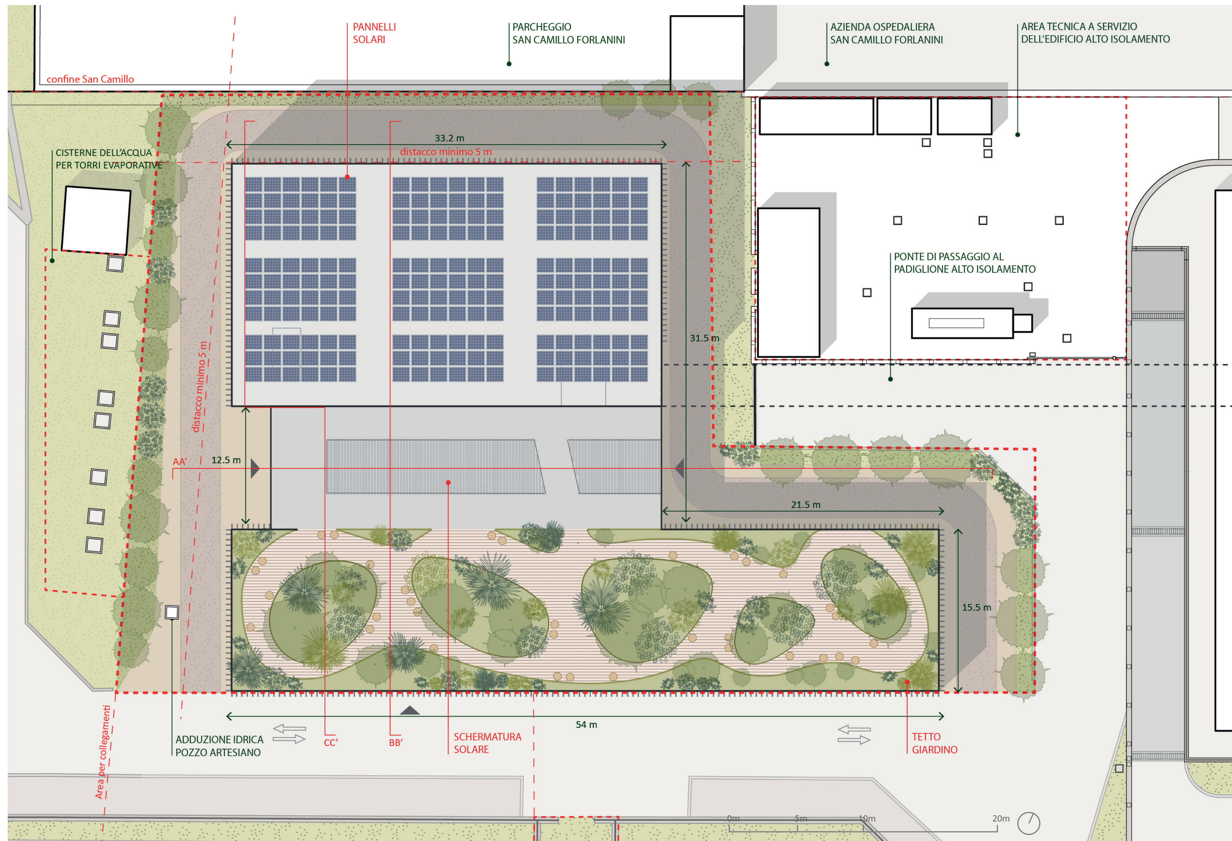
Planimetria generale copertura
