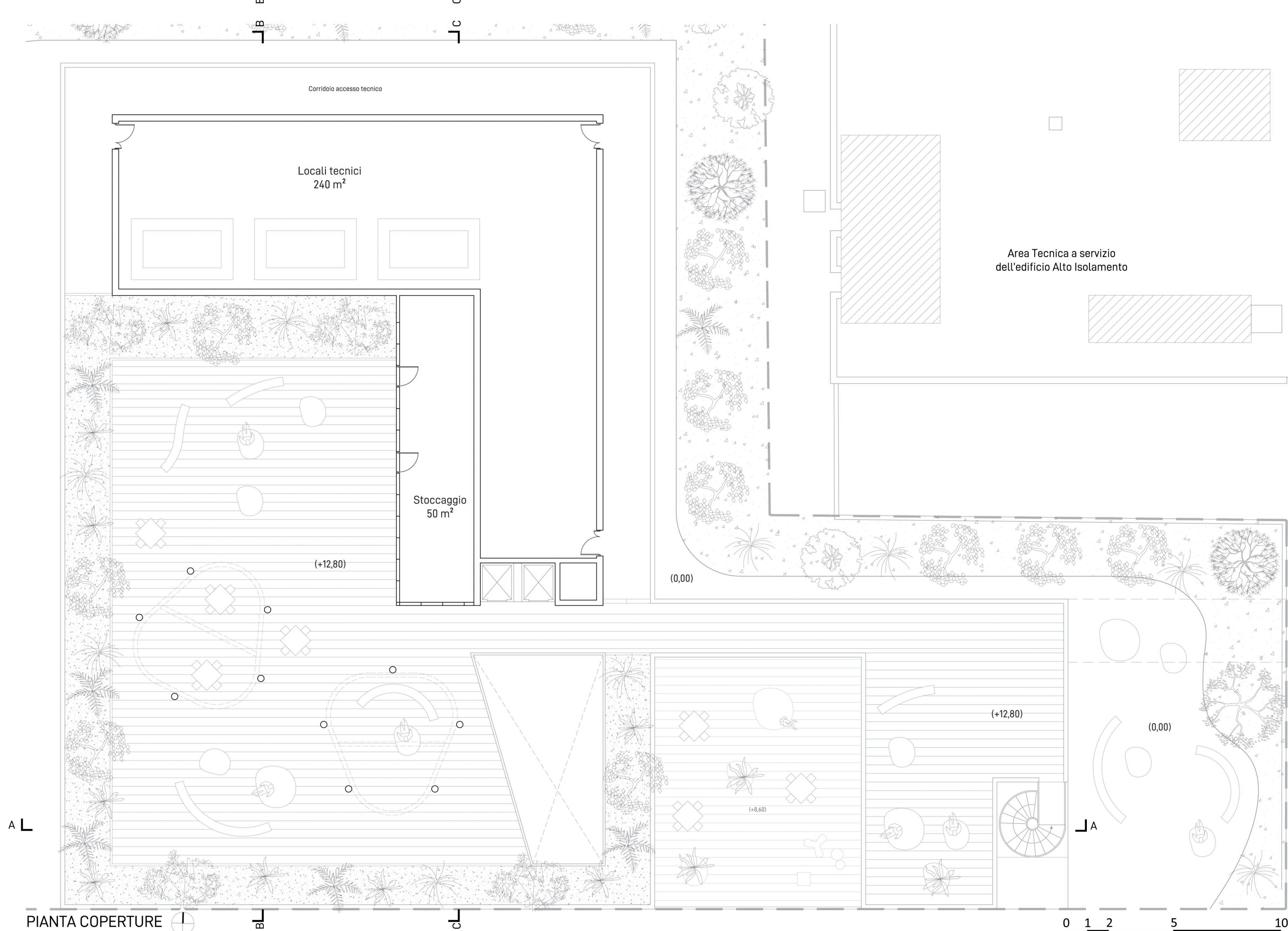
PIANTA COPERTURE
