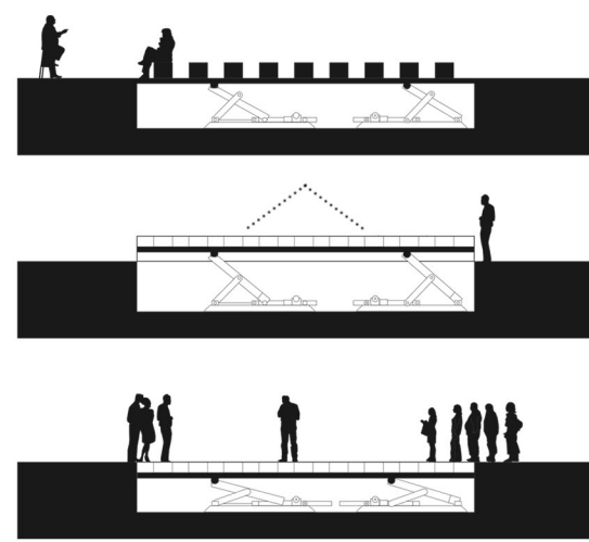
Particolare costruttivo - 1:40
