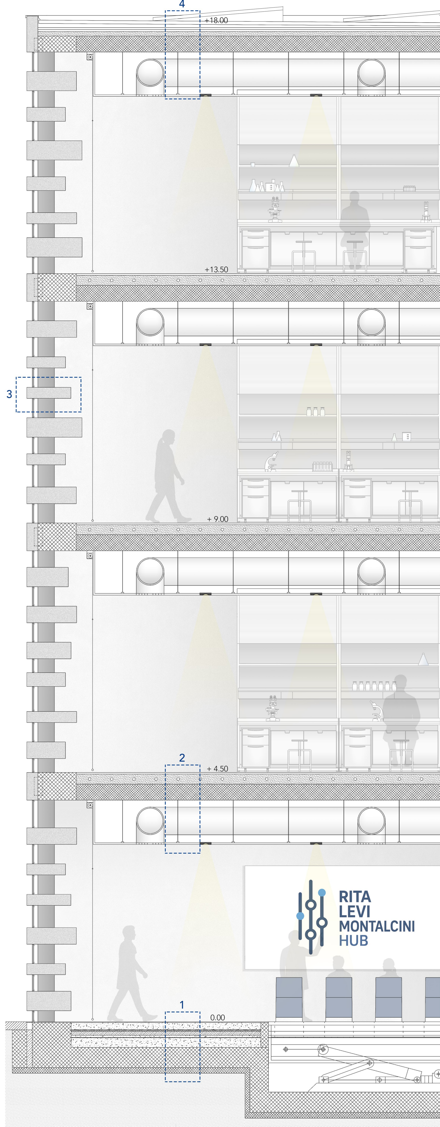
Particolare costruttivo - 1:40
