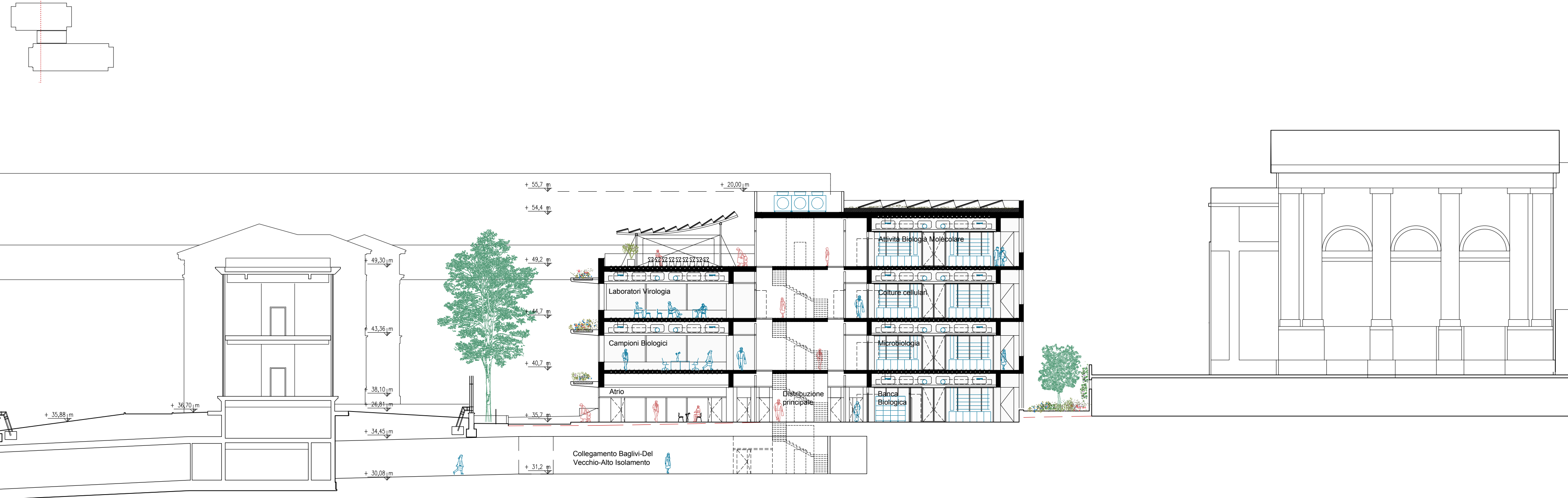
SEZIONE TRASVERSALE SCALA 1:250
