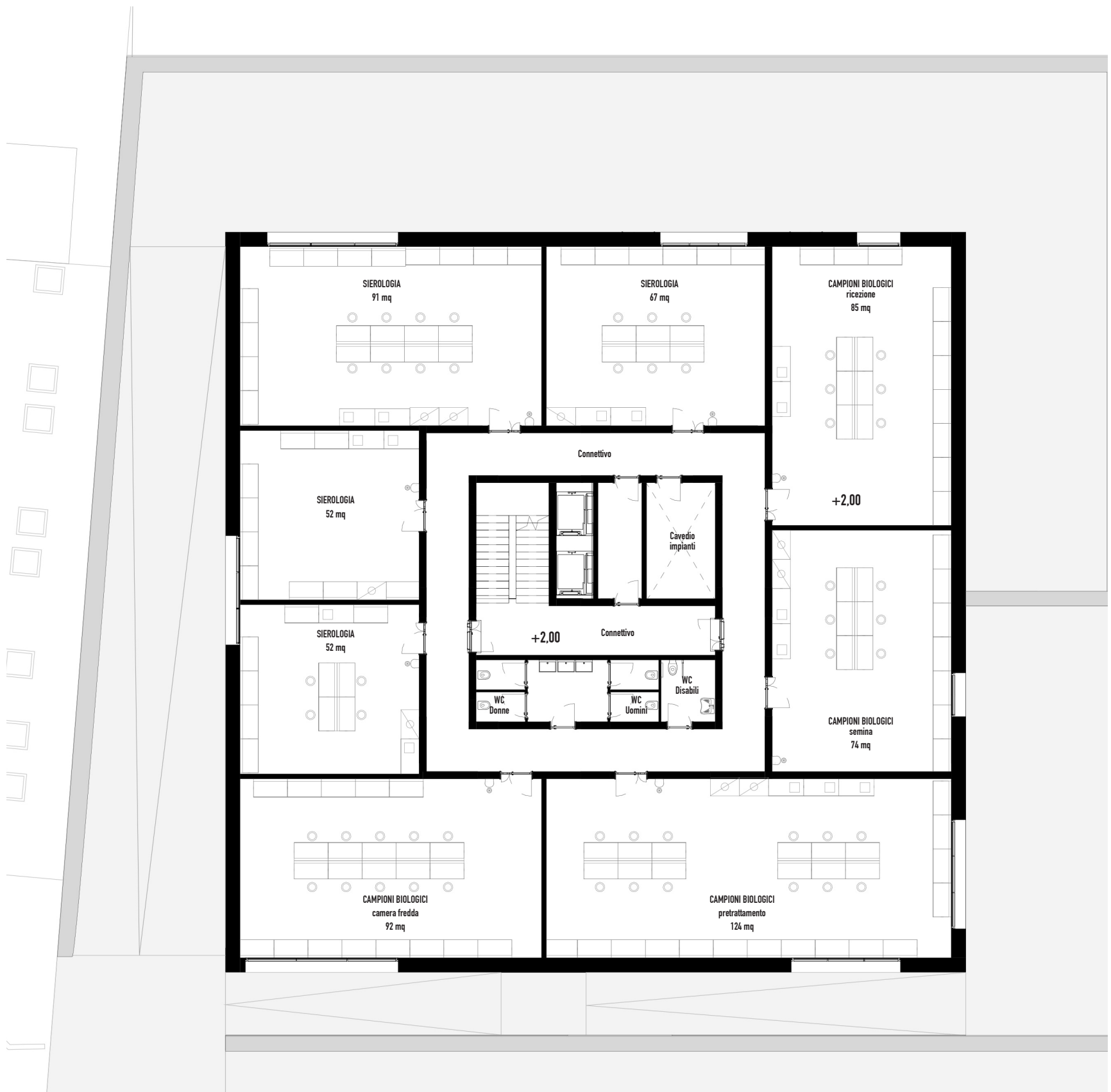
PIANO PRIMO 1:200 (+2,00)
