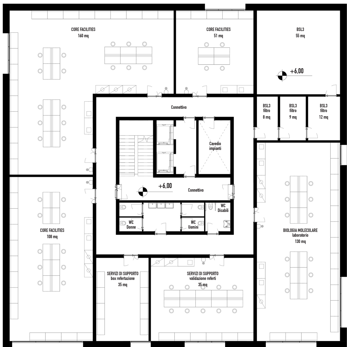
PIANO SECONDO 1:200 - (+6,00)
