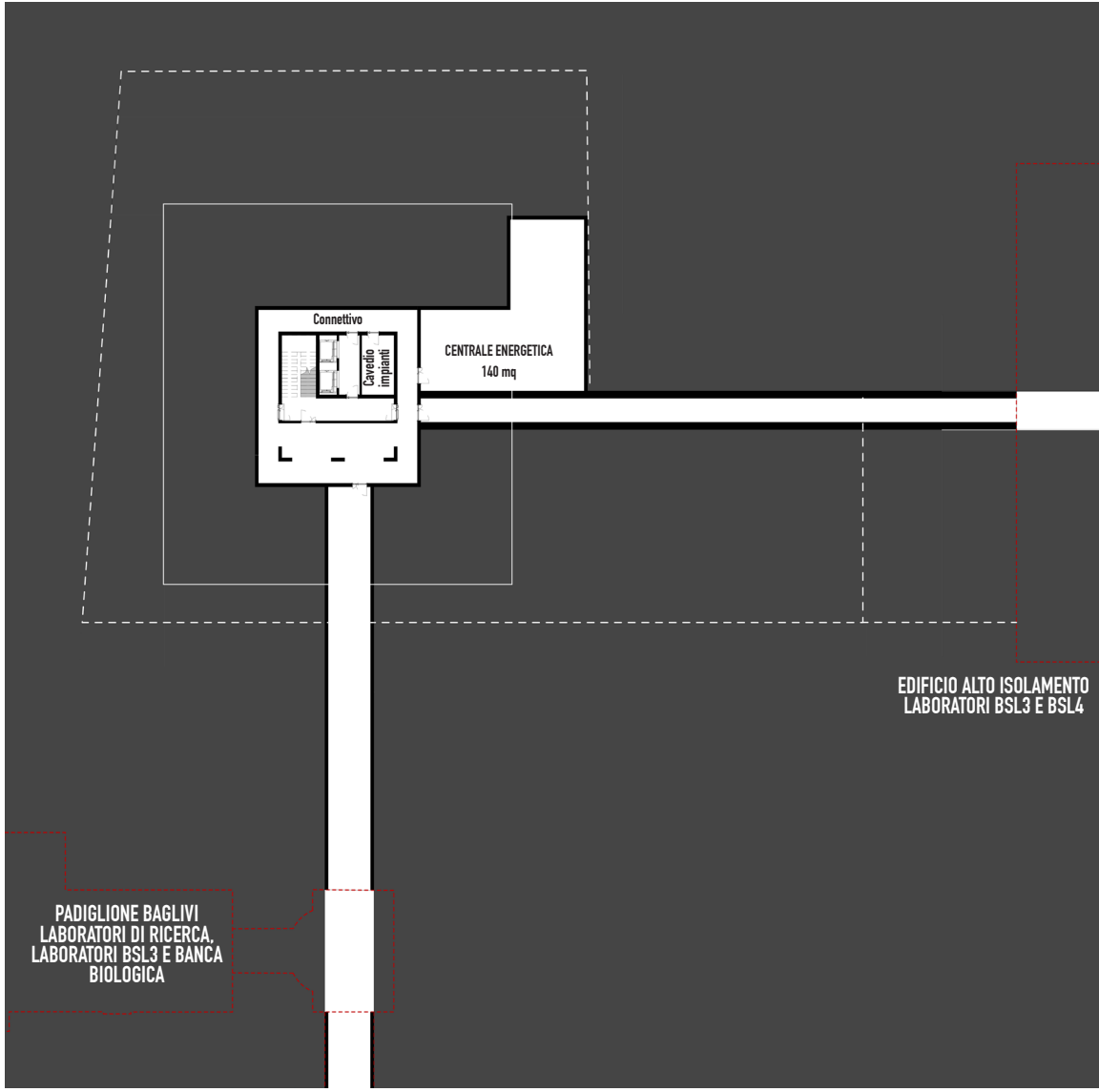
SCHEMA PIANO INTERRATO - (-6,00)
