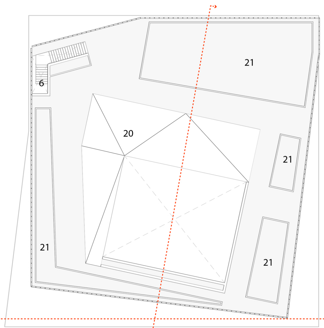
Pianta Copertura
