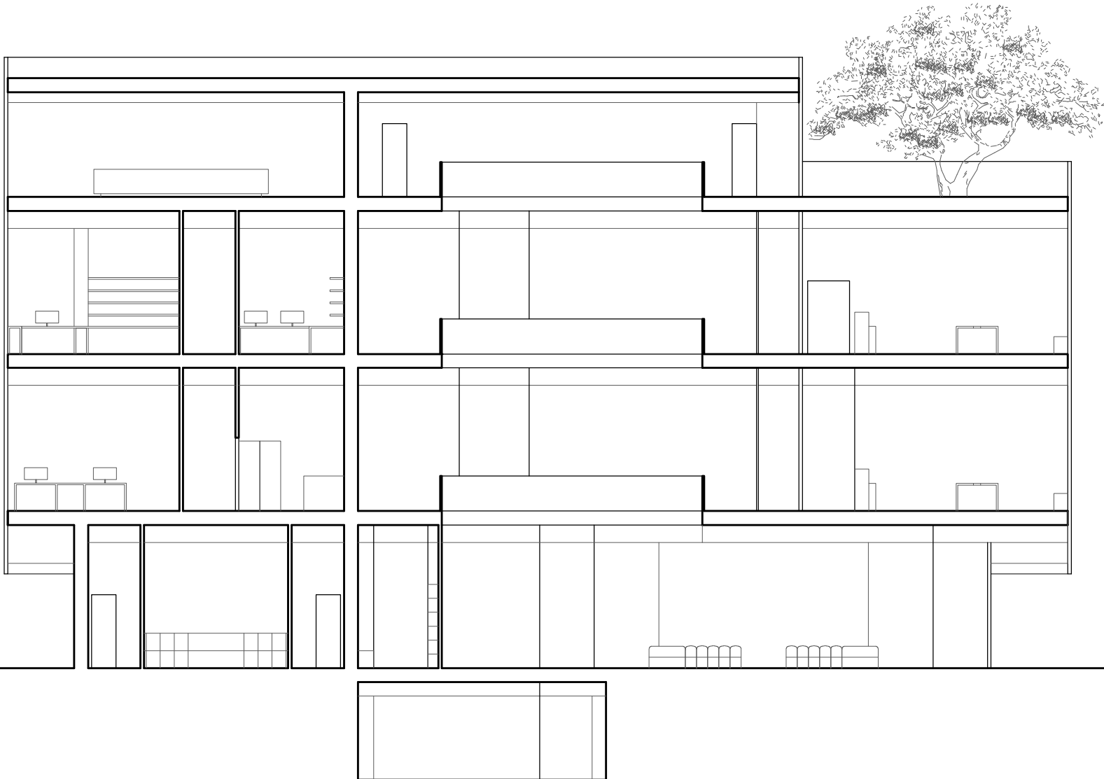
SEZIONE CC' scala 0 1 5
