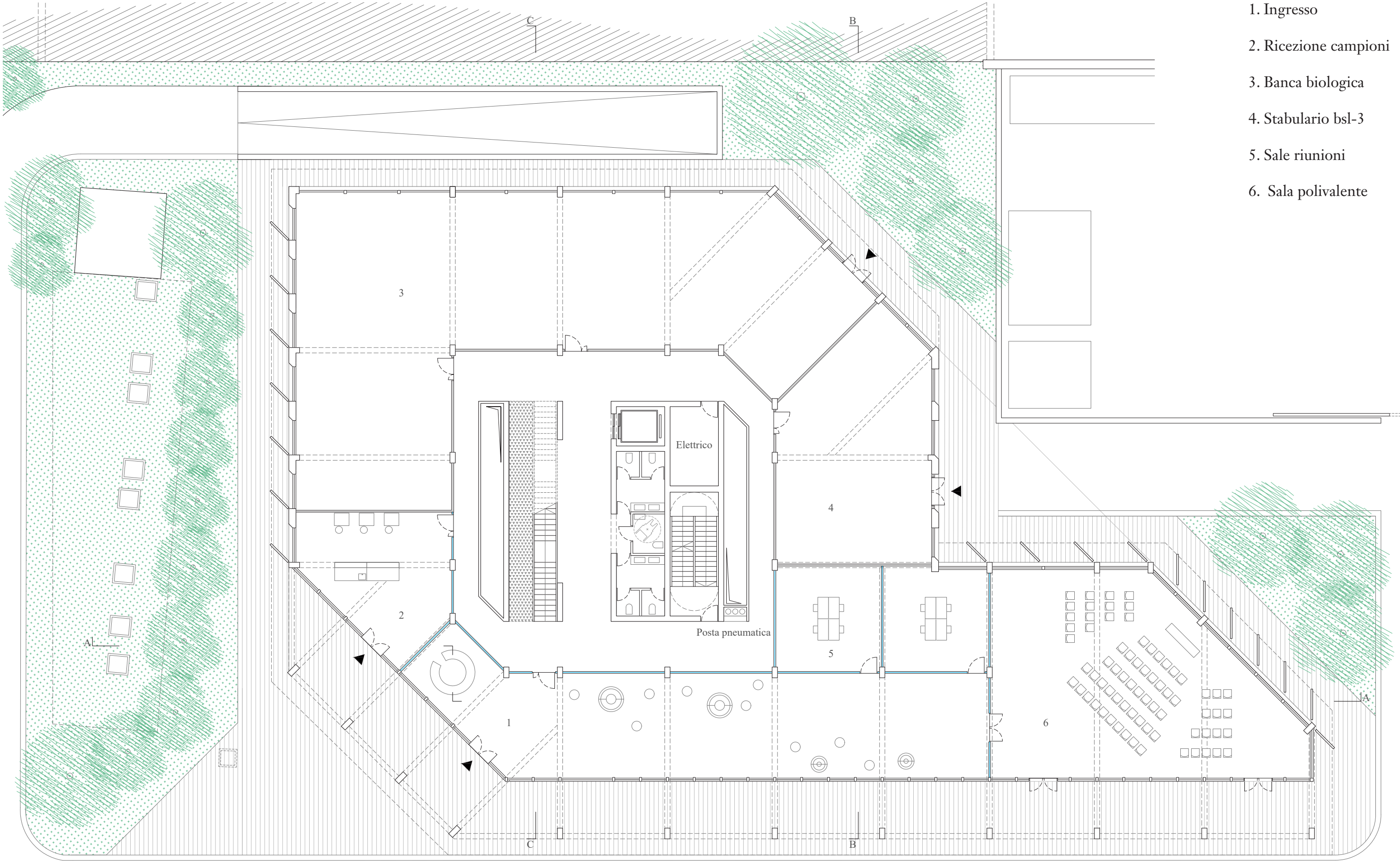
Pianta piano terra | 1:200
