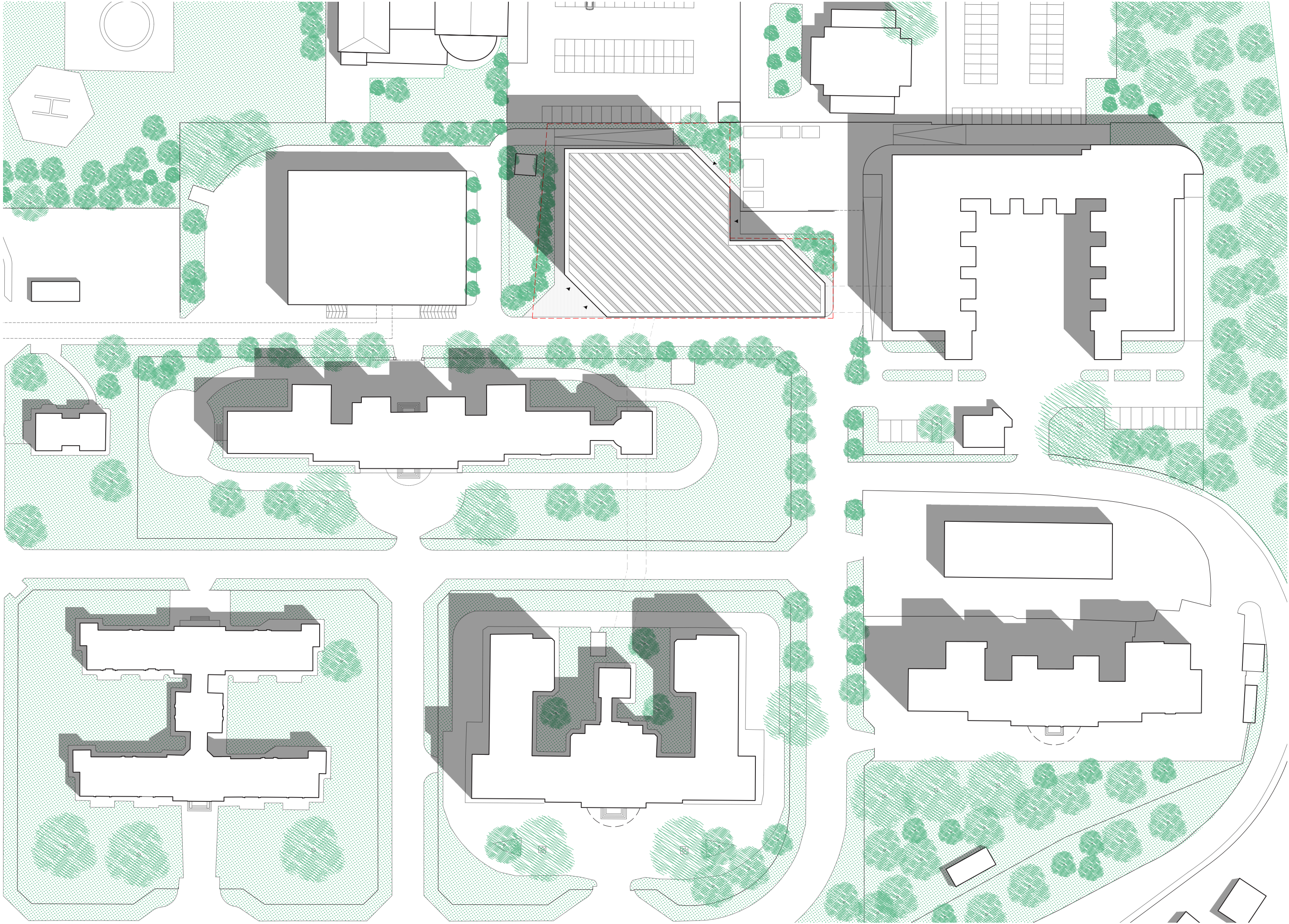
Planivolumetrico | 1:750
