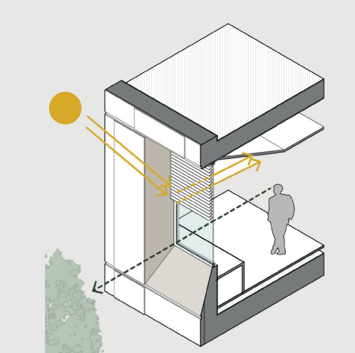
Finestre su parete massiva edificio
