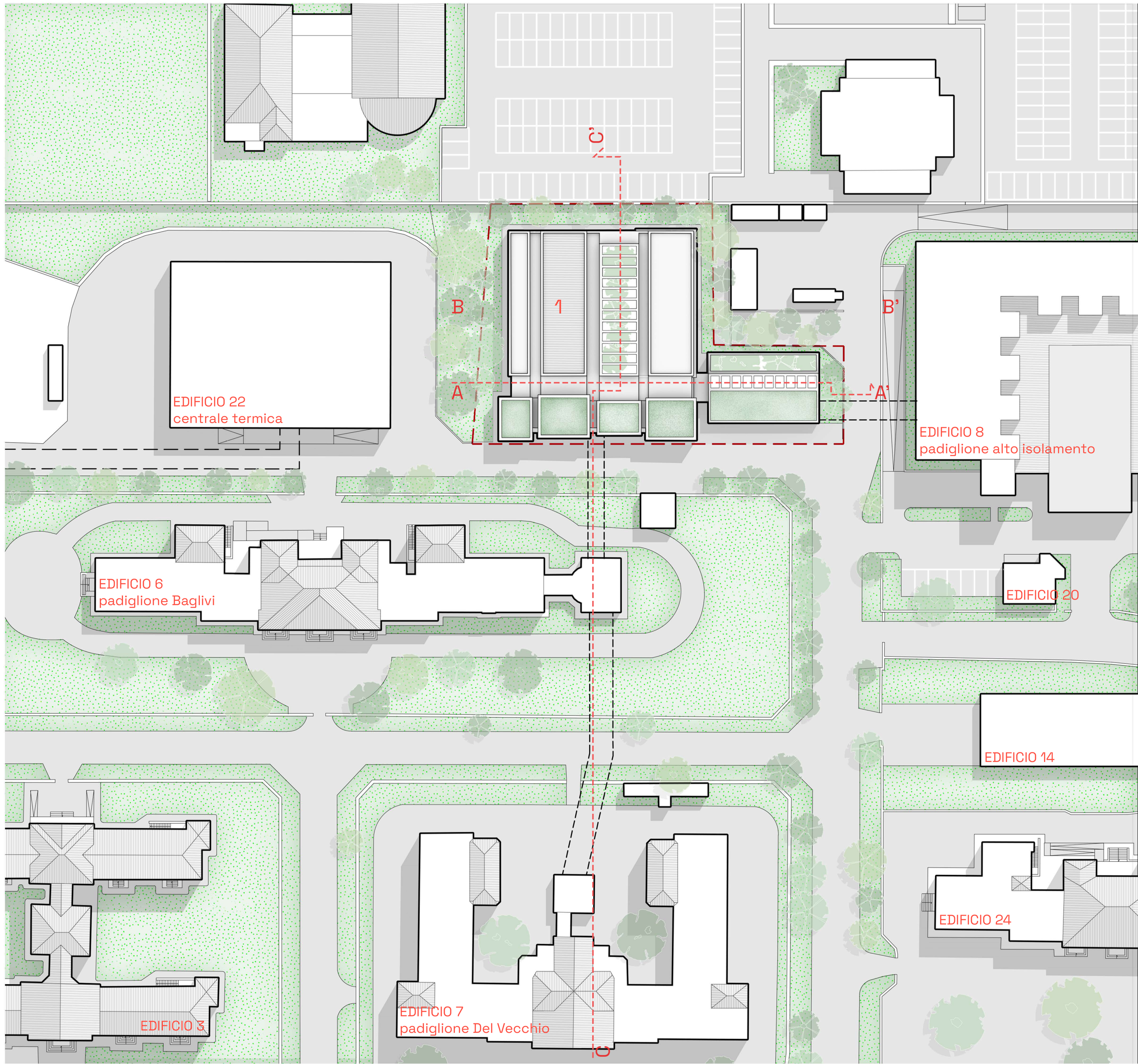
planovolumetrico scala 1:500
